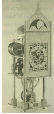
Osmanlı bilgini Takiyeddin'in 1559 yılında yaptığı mekanik saat. Modelimiz Saatlere Dair kitabındaki resim ve tariflere göre yapılmıştır (Katalog, III, 119; no. B 3.14)
