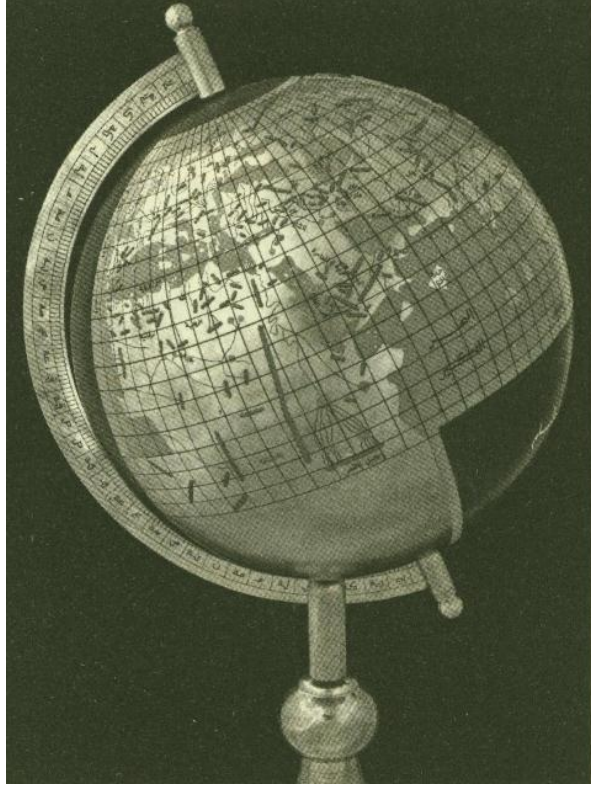
Yer küresi
